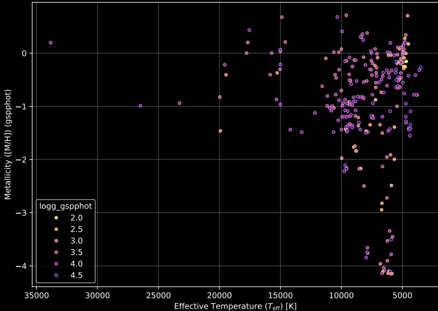
APOGEE DR17 Field: [288-01-C] Stellar Population Parameters (n= 263)
