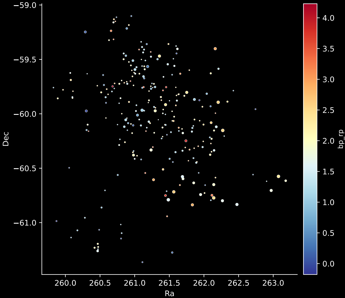
APOGEE DR17 Field: [288-01-C] Stars: 263
